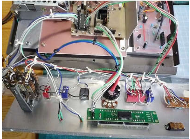
(14) 配線完了
