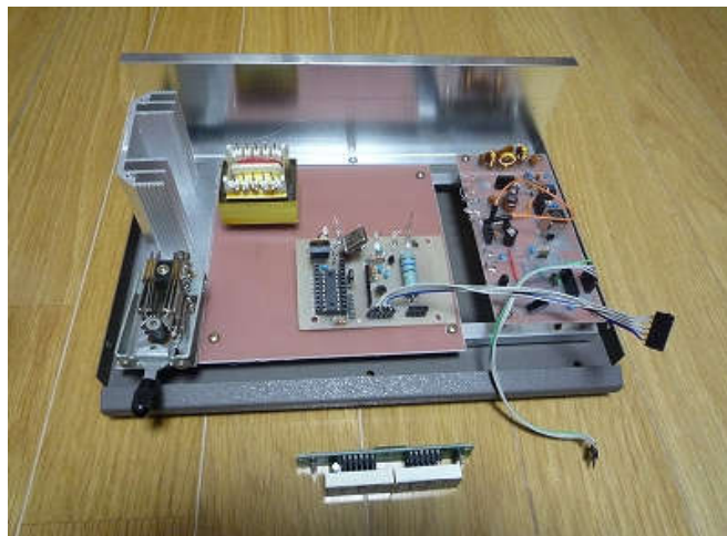
(2) 配置検討
